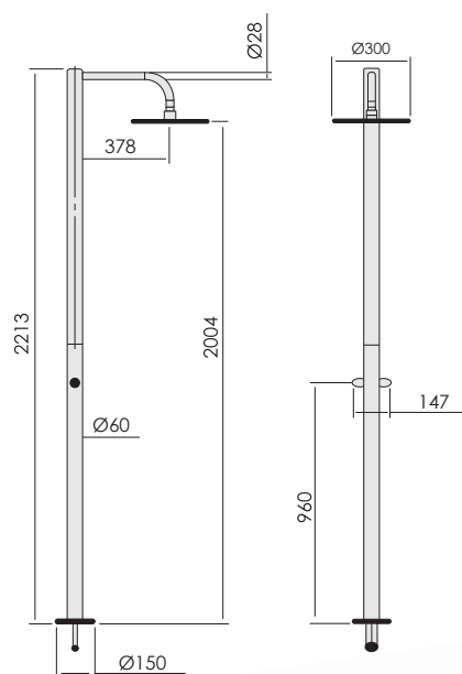
Colonne de douche LUX & COLOUR
